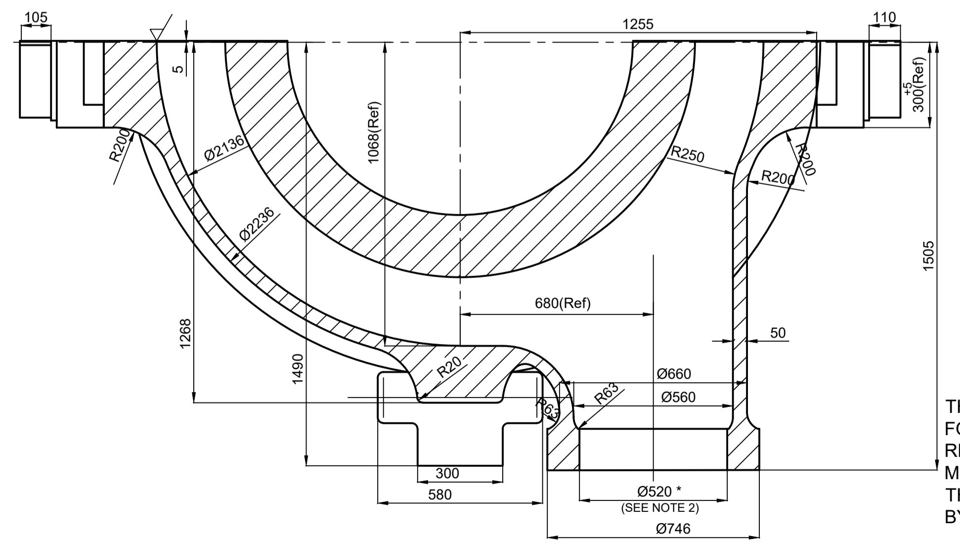
SECTION A5-A5
