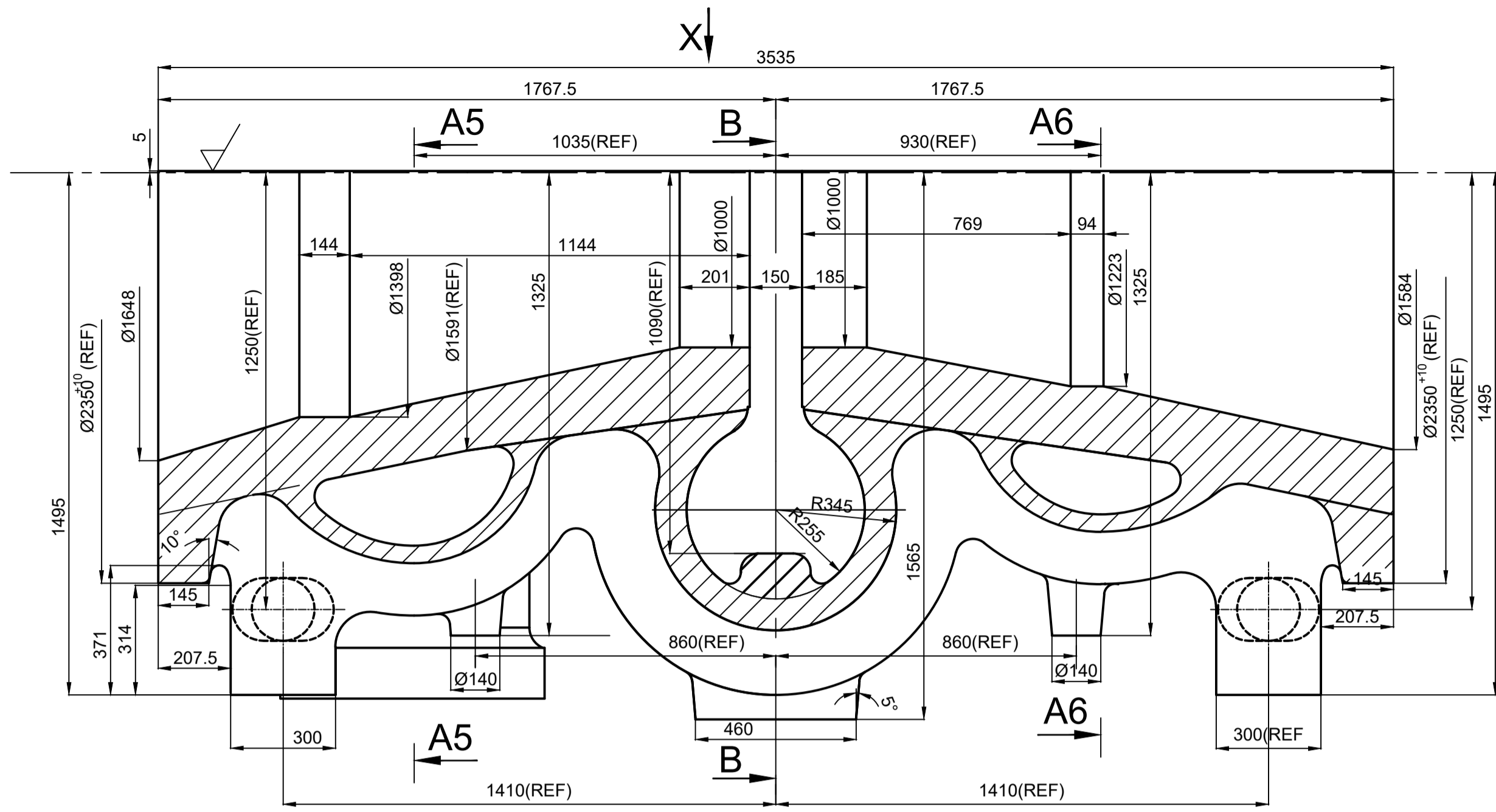
SECTION A-A
